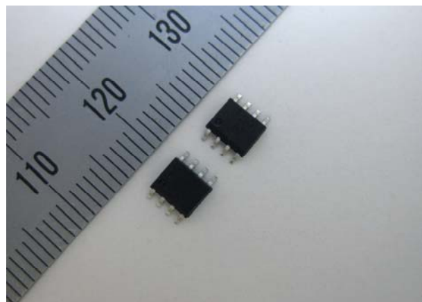
▲XC9270/XC9271 シリーズ SOP-8FD (4.9 x 6.0 x h1.55mm)
