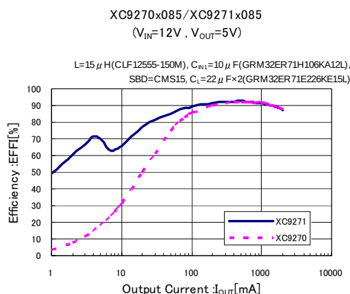
▲XC9270/XC9271 シリーズ特性例
