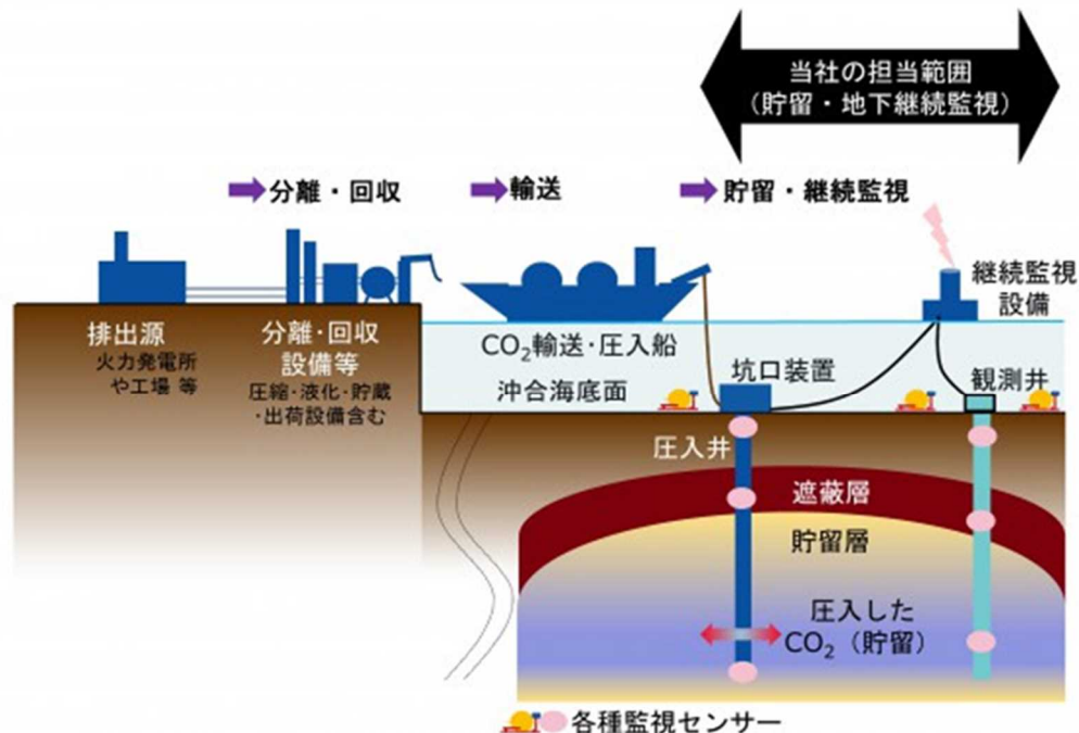
沖合海底下へのCO 2 地下貯留を想定した一貫実証実証試験イメージ図
